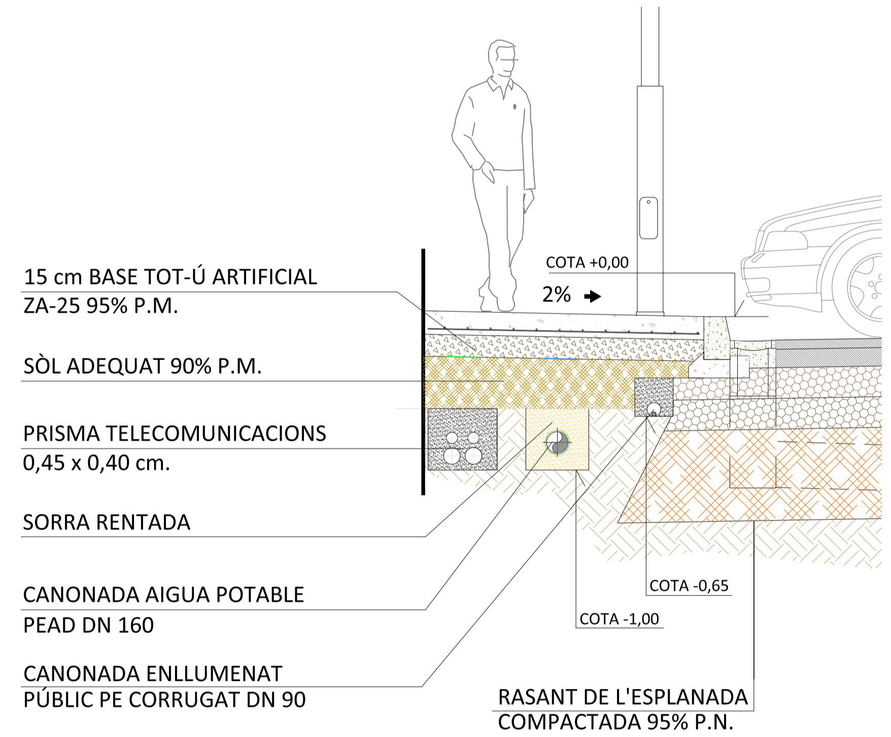
DETALL PAS DE RASA E= 1/25
