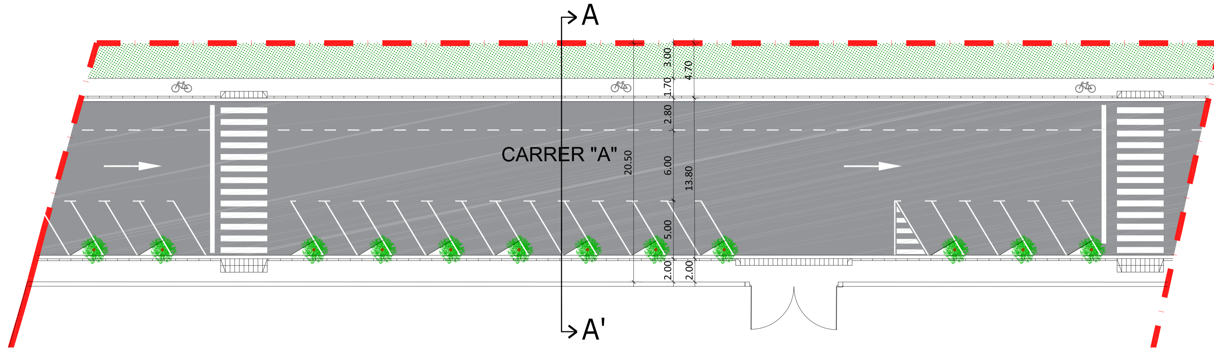
PLANTA GENERAL. CARRER A E= 1/200
