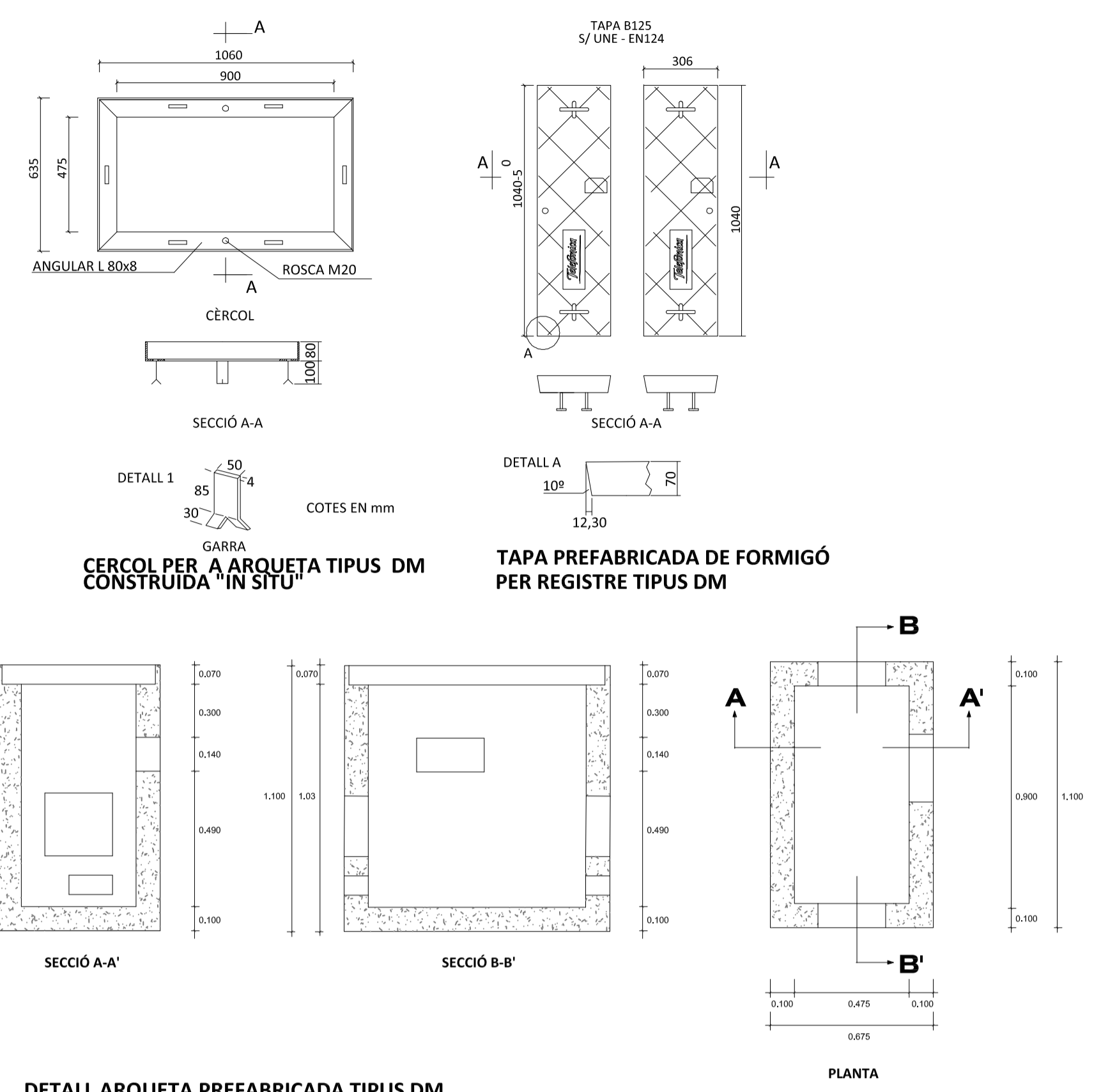
DETALL ARQUETA PREFABRICADA TIPUS DM E= 1/20
