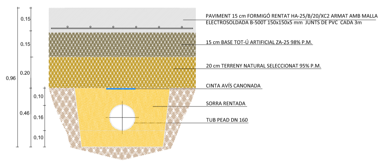
DETALL RASA CANONADA DN 160 E= 1/15
