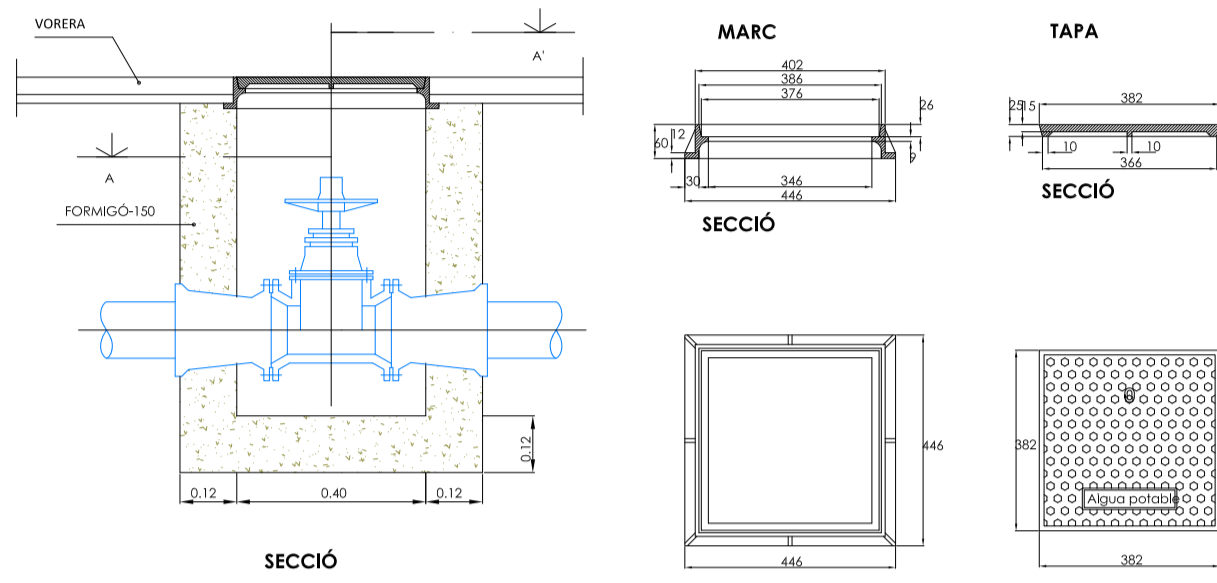
MARC I TAPA DE FOSA 0.40 x 0.30 E= 1/20
