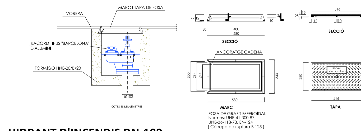
HIDRANT D'INCENDIS DN-100 E= 1/20
