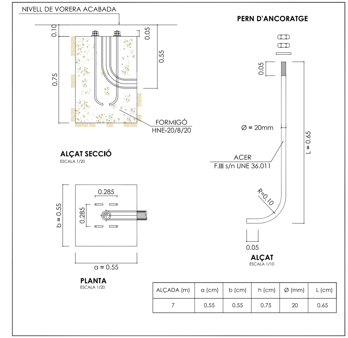
DETALL FONAMENTACIÓ BÀCUL E= 1/20
