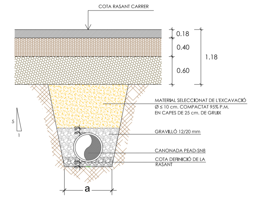
DETALL RASA PAS CANONADA E= 1/50
