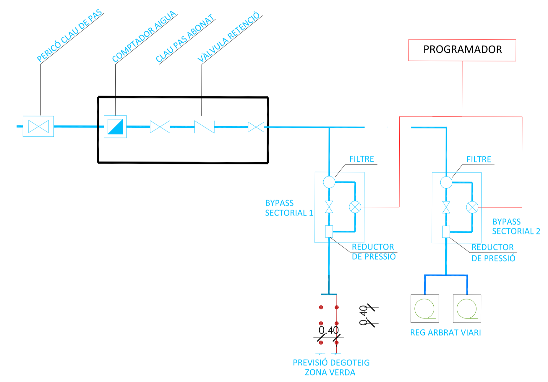
ESQUEMA XARXA DE REG
