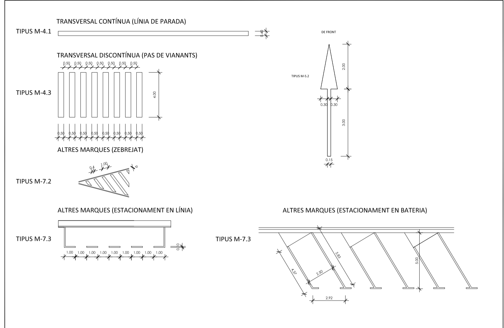
SENyalITZACIÓ HORIZONTAL E= 1/200
