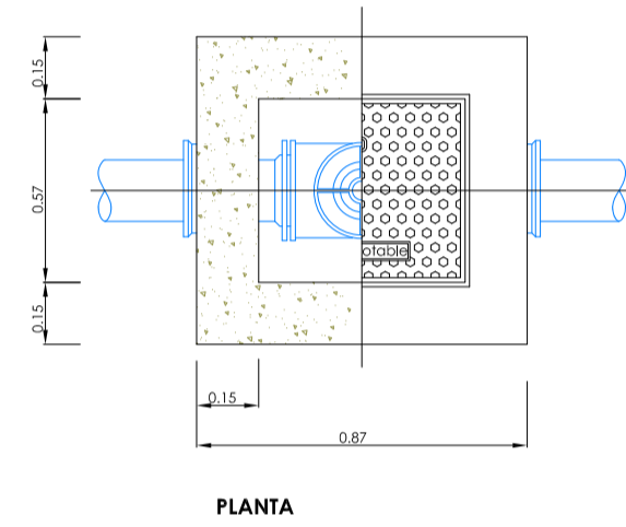
ARQUETA DE REGISTRE E= 1/20
