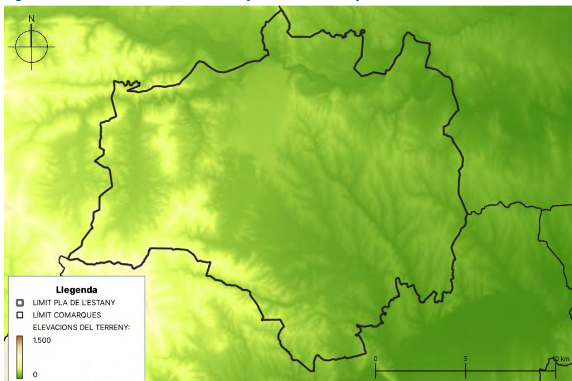
Figura 2.2 Model d'elevacions del terreny del Pla de l'Estany
