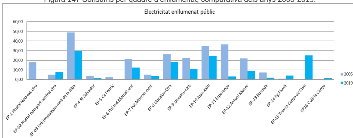
Figura 147 Consums per quadre d'enllumenat, comparativa dels anys 2005-2019.
