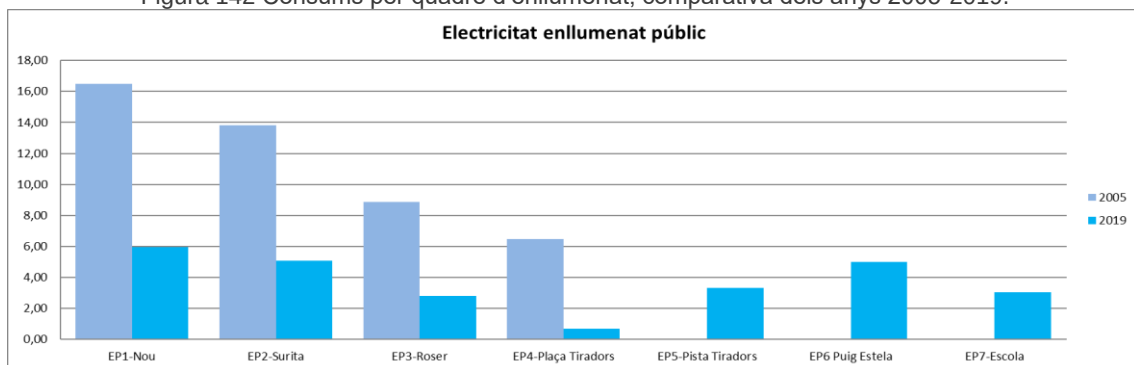
Figura 142 Consums per quadre d'enllumenat, comparativa dels anys 2005-2019.
