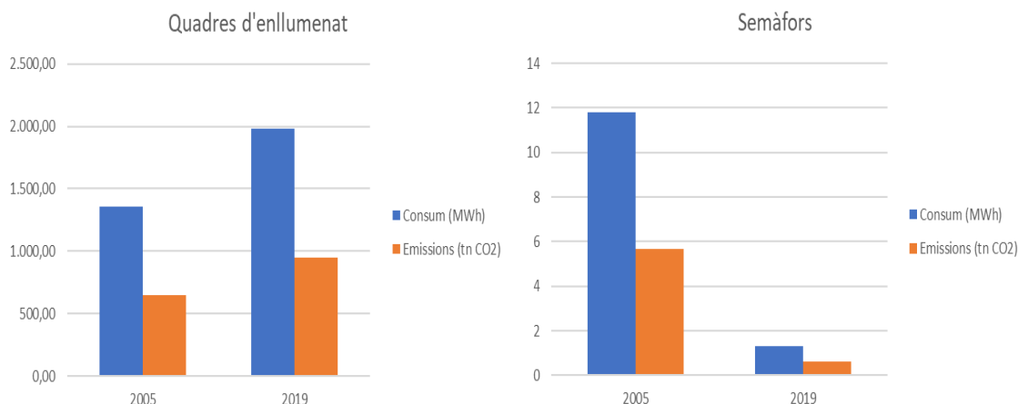
Figura 137 Consums i emissions per quadre d'enllumenat i semàfors, comparativa dels anys 2005-2019.
