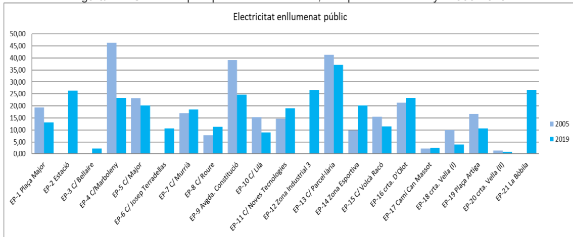
Figura 141 Consums per quadre d'enllumenat, comparativa dels anys 2005-2019.
