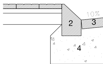
SECCIÓ DETALL B E:1/20
