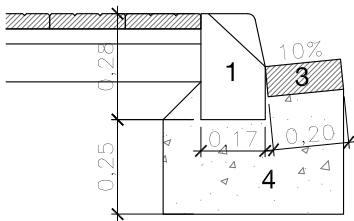
SECCIÓ DETALL A E:1/20
