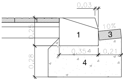
SECCIÓ DETALL A E:1/20
