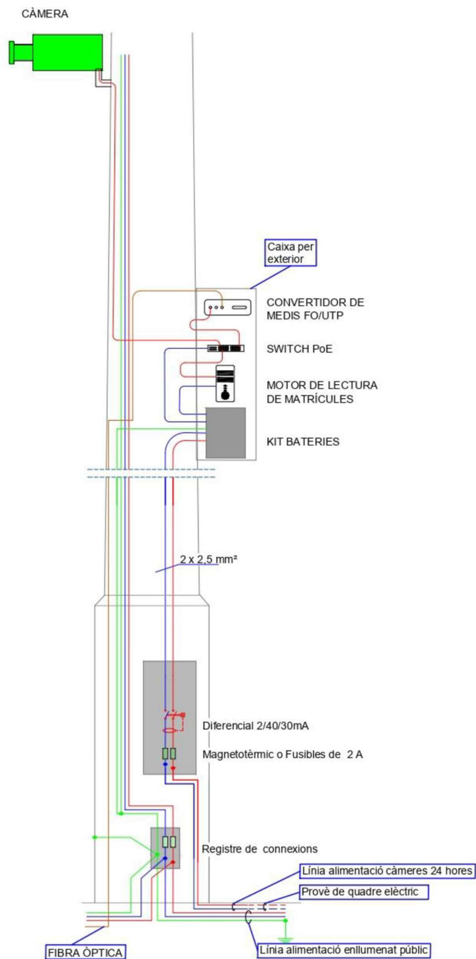
Esquema de connexions en fanal de 1 càmera
