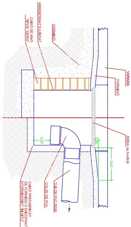
EMBORNAL SIFÒNIC AMB REIXA figura 13 e:1/20
