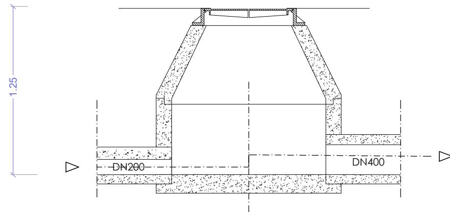
SECCIO A-A'
