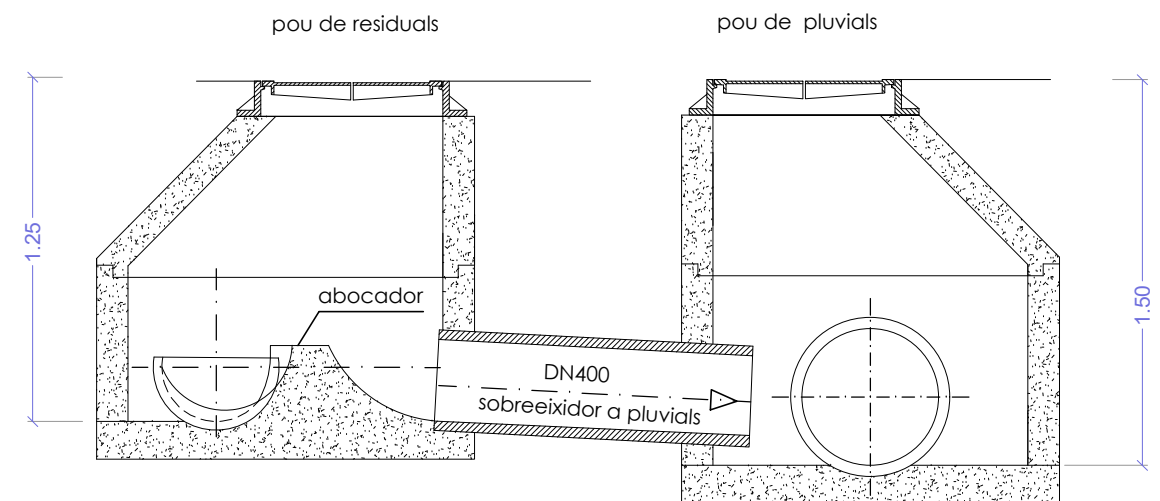
SECCIO B-B'
