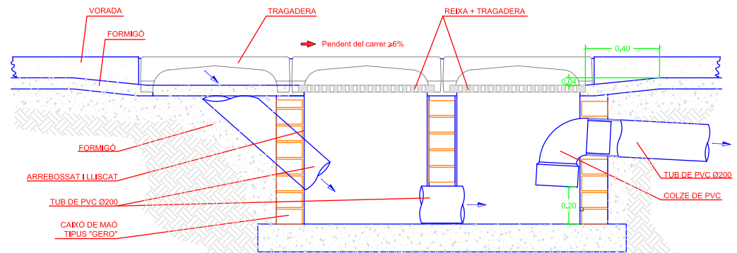
MUNTATGE D'EMBORNAL SIFÒNIC AMB 2 REIXES i 3 "BÚSTIES" figura 16 e:1/20
