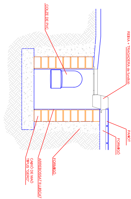
EMBORNAL SIFÒNIC AMB REIXA i "BÚSTIA" (secció transversal) figura 12.2 e:1/20
