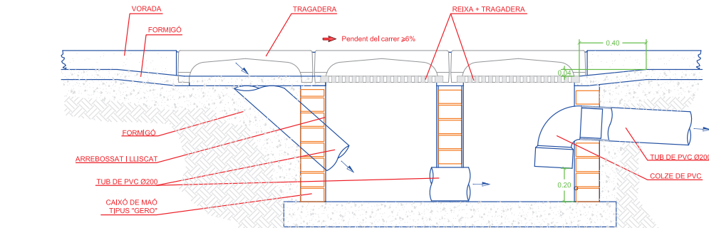
MUNTATGE D'EMBORNAL SIFÒNIC AMB 2 REIXES I 3 "BÚSTIES" figura 16 e:1/20
