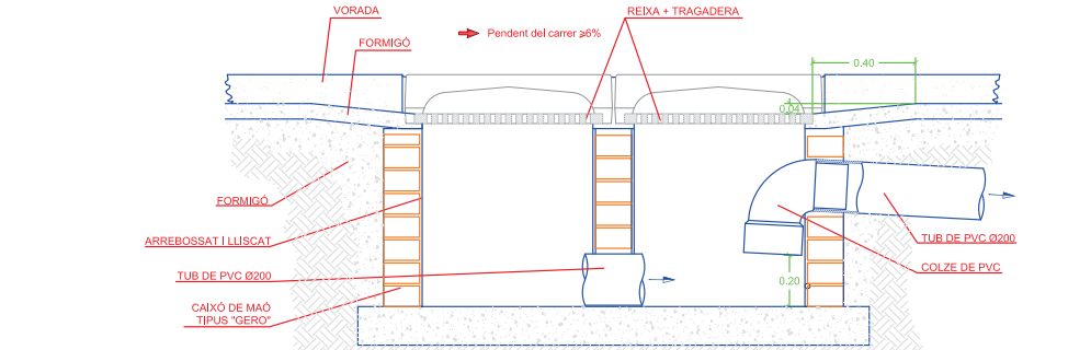
MUNTATGE D'EMBORNAL SIFÒNIC AMB 2 REIXES I 2 "BÚSTIES" figura 14 e:1/20
