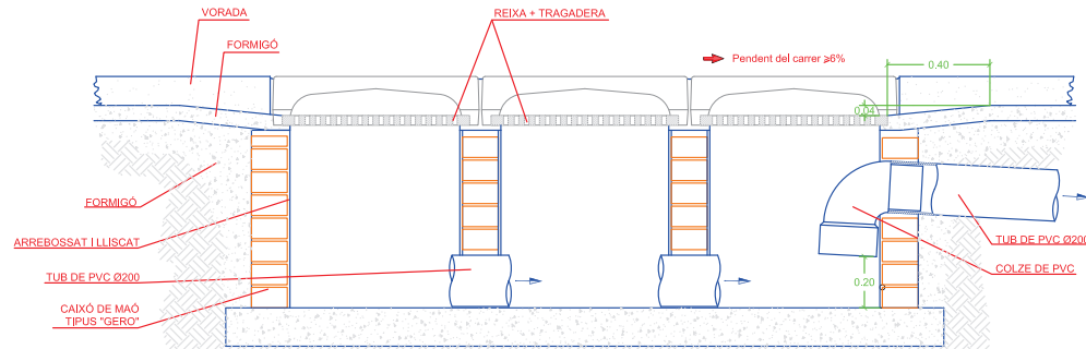
MUNTATGE D'EMBORNAL SIFÒNIC AMB 3 REIXES I 3 "BÚSTIES" figura 15 e:1/20
