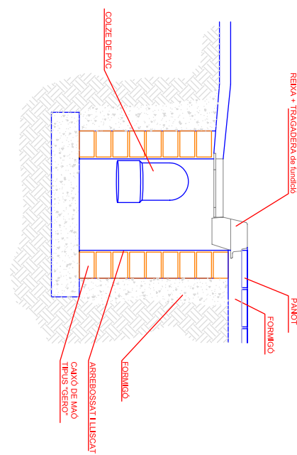
EMBORNAL SIFÒNIC AMB REIXA i "BÚSTIA" (secció transversal) figura 12.2 e:1/20
