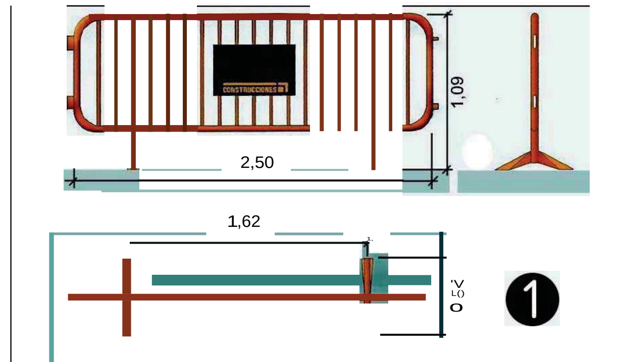
11. tanca provisionalobra
