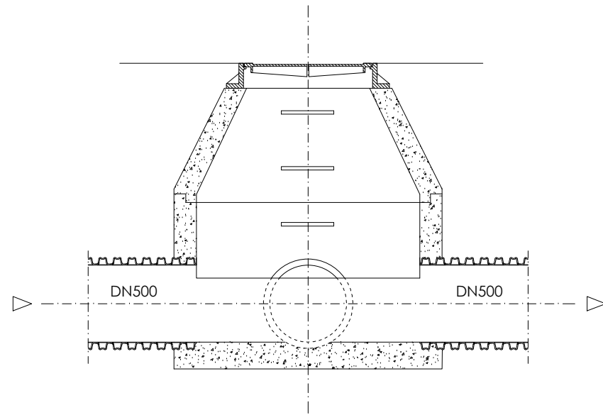
SECCIO A-A'
