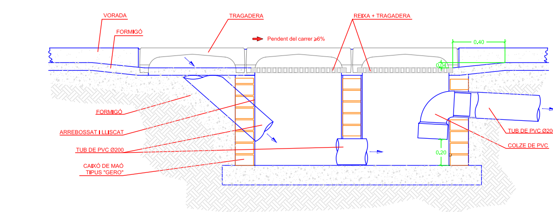
MUNTATGE D'EMBORNAL SIFÒNIC AMB 2 REIXES i 3 "BÚSTIES" figura 16 e:1/20
