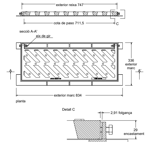
Reixa d'embornal
