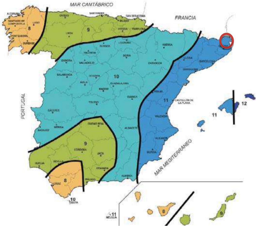
La zona d'estudi es troba en la regió de torrencialitat I_1/I_d=11
