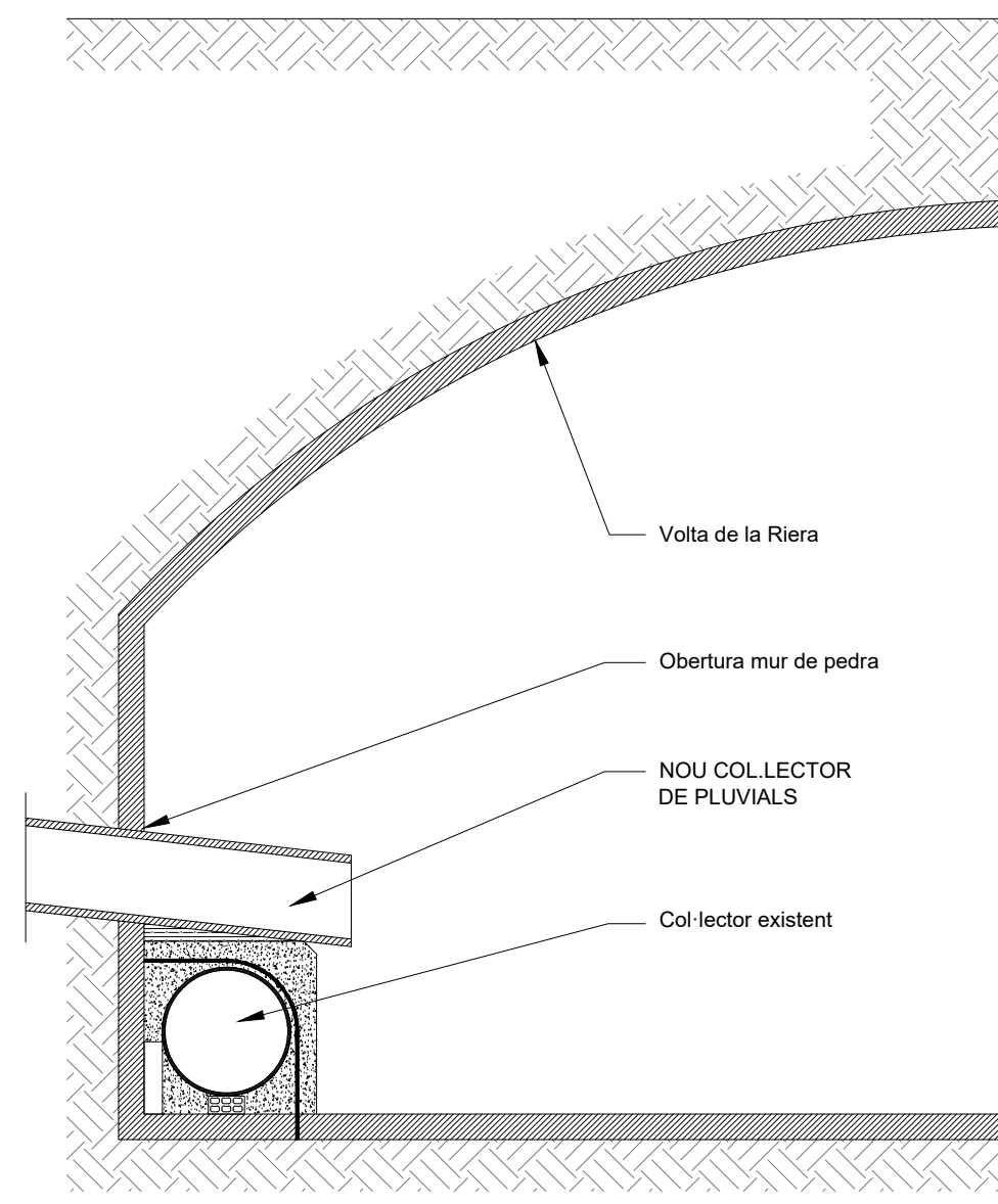
secció transversal
