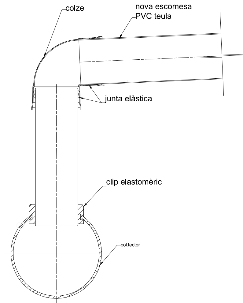
SECCIÓ A-A'
