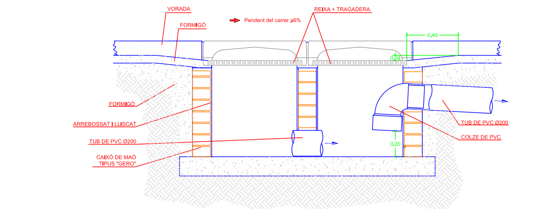
MUNTATGE D'EMBORNAL SIFÒNIC AMB 2 REIXES i 2 "BÚSTIES" figura 14 e:1/20
