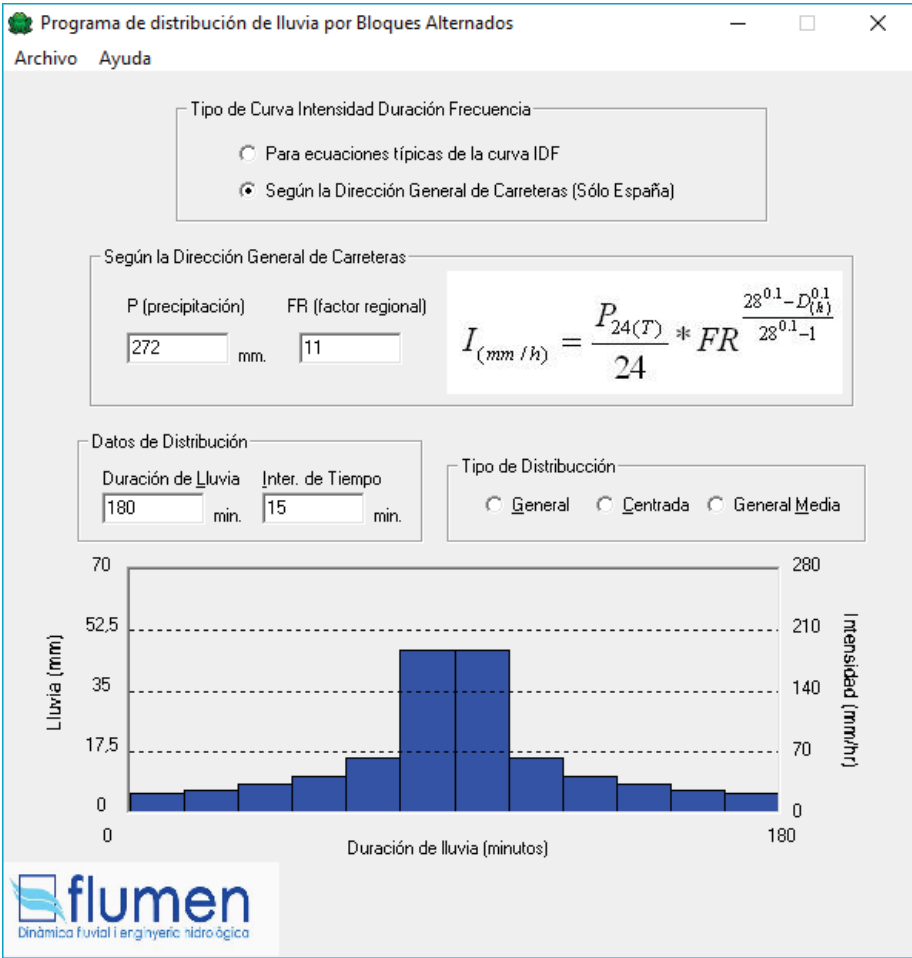
Hietograma optingut amb el programa "programa de distribución de lluvia por el método de los bloques alternados" versió 2015
