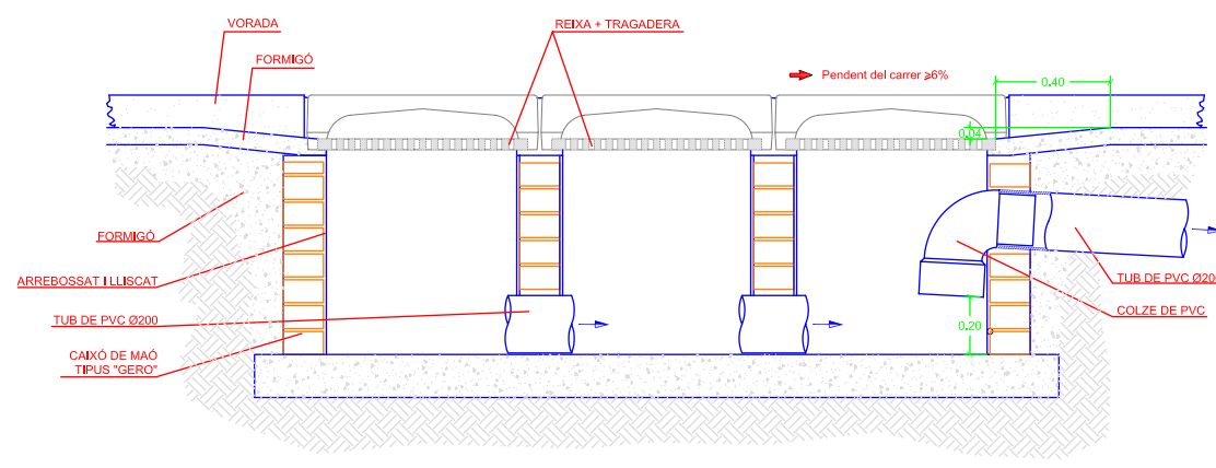
MUNTATGE D'EMBORNAL SIFÒNIC AMB 3 REIXES i 3 "BÚSTIES" figura 15 e:1/20
