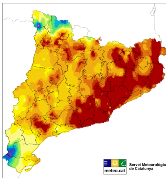
ÍNDEX DE PRECIPITACIÓ ESTÀNDARD IPE24
