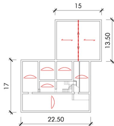
Planta Soterrani
