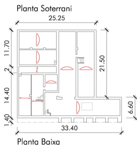
Planta Baixa
