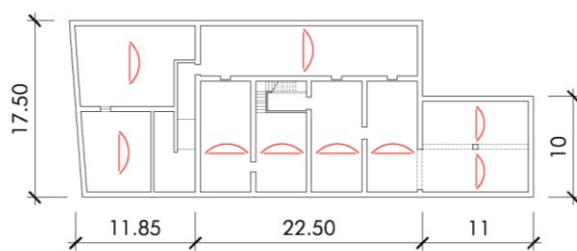
Planta Baixa
