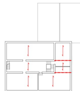
Planta Primera
