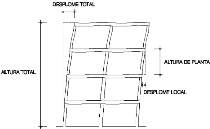
Figura 4.1 Desplomes
