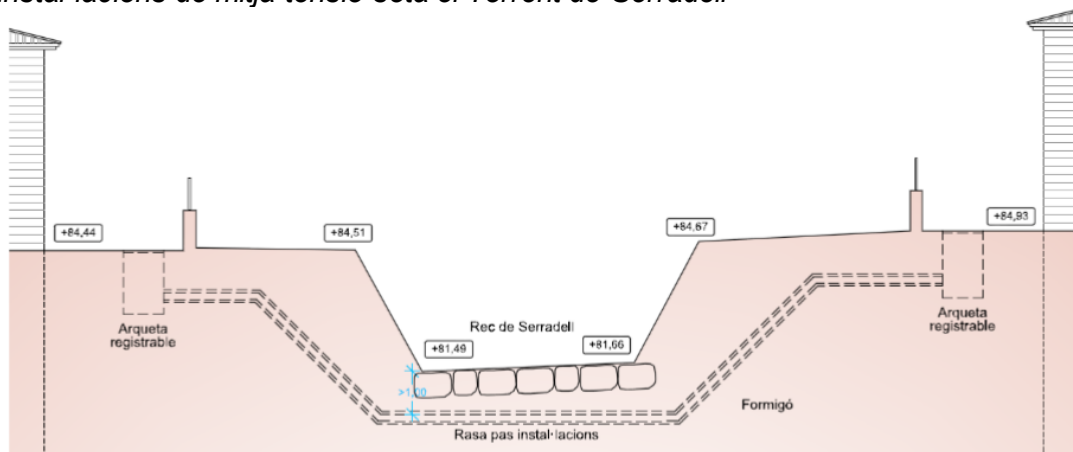
PERFIL TRANSVERSAL TORRENT
