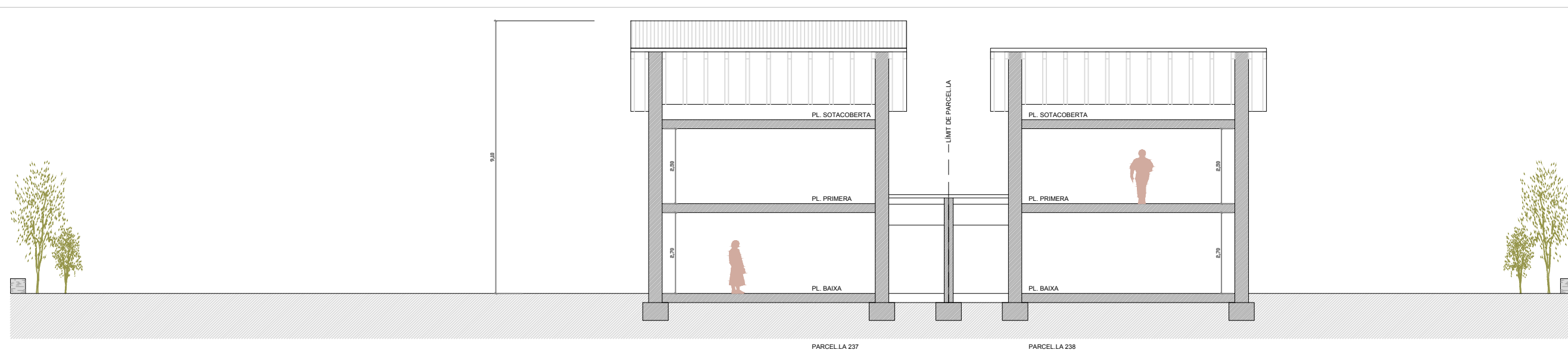
SECCIÓ TRANSVERSAL PARCEL.LA 238
