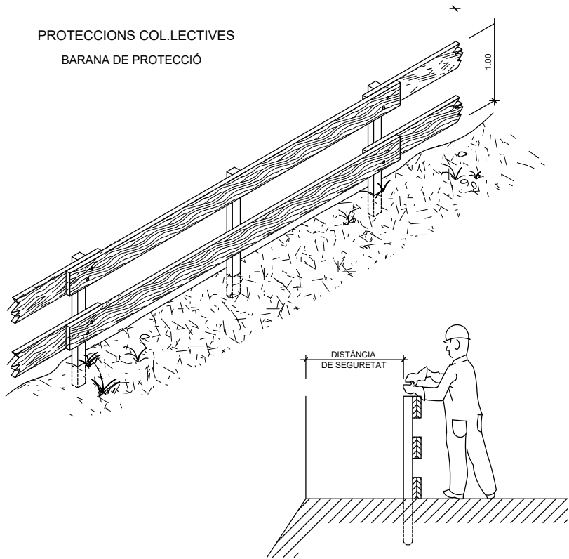
BARANA AMB SUPORT TIPUS "SARGENTO"
