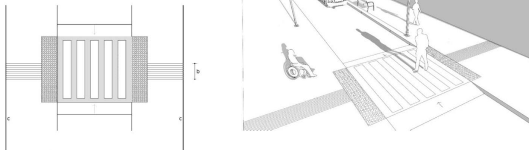
Aplicació del paviment tàtil indicador en creuament amb pas de vianants elevat (Guia d'accessibilitat en espais públics urbanitzats segons OM TMA/851/2021)
