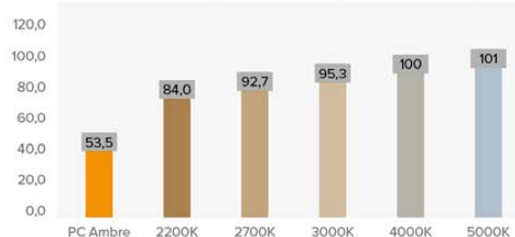
Relació Eficiència (%) lm/W - Temperatura de Color (K)
