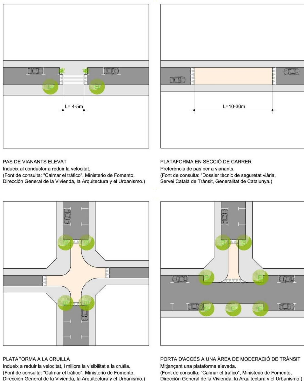
Figura 23. Elevacions a la calçada
