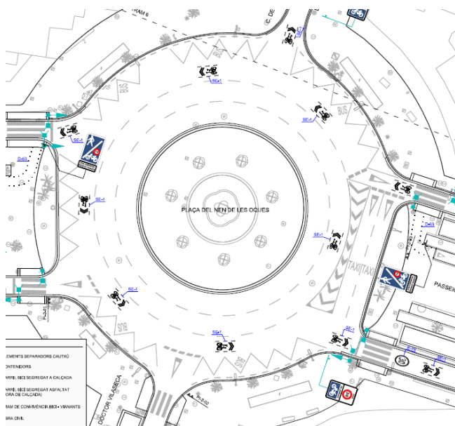
Figura 49. Exemple de configuració de circulació en calçada de bicicletes en rotonda (pictogrames)
