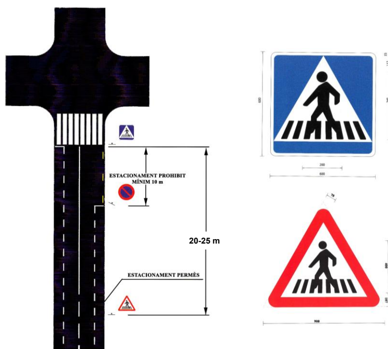
Figura 44. Senyalització vertical d'un pas de vianants
