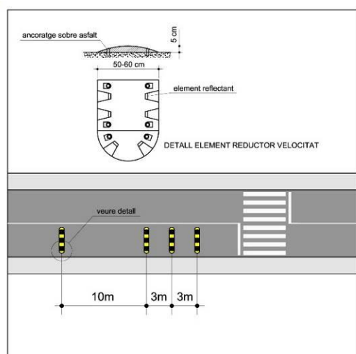
Figura 24. Figura 1 Elements transversals de reducció de velocitat
