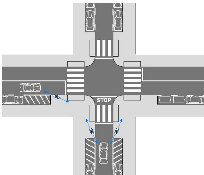
Figura 37. Exemple d'aplicació d'orelles als passos de vianants
