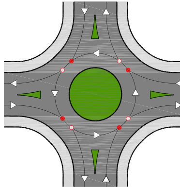
Figura 26. Punts de conflicte en una rotonda
