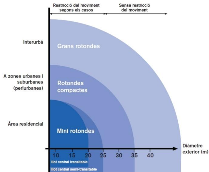
Figura 52. Dimensionament de les rotondes
