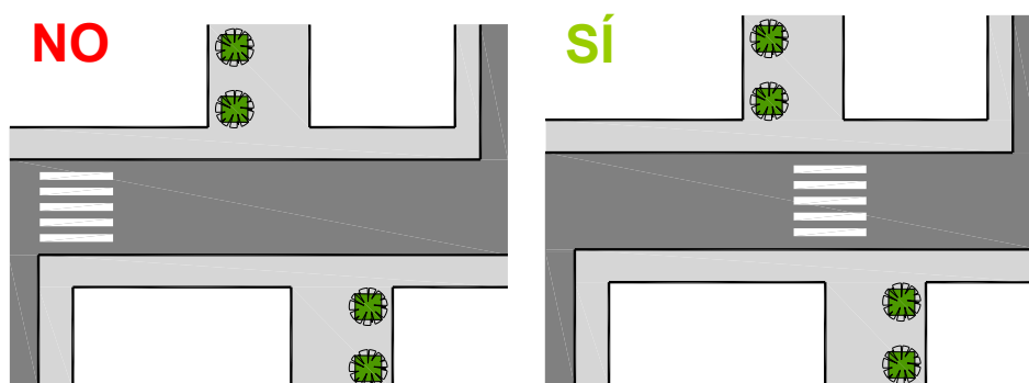
Figura 42. Recomanacions d'ubicació de passos de vianants
