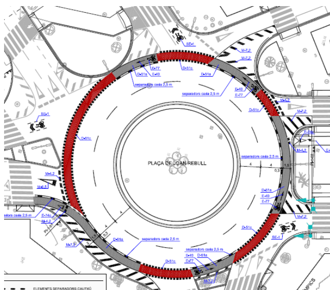
Figura 48. Exemple de configuració de carril pedalable segregat en rotonda
