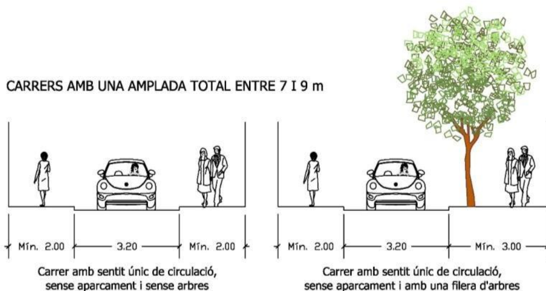
Figura 17. Seccions per a carrers amb amplada de 7 a 9 metres
