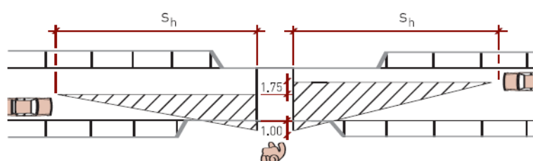
Figura 35. Paràmetres pel càlcul de les distàncies de visibilitat dels vianants
