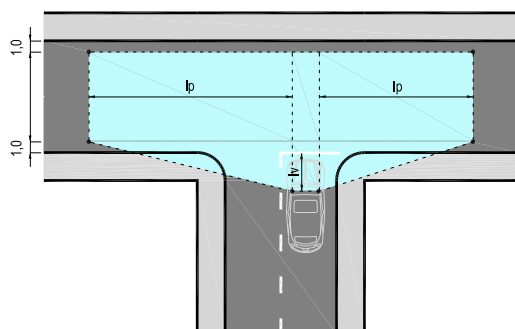
Figura 30. Àrea de visibilitat en interseccions en T
