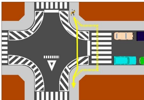
Figura 33. Ubicació correcta de pas de vianants. Possible ocupació del pas i restricció de la visibilitat
