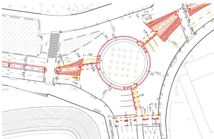
Figura 50. Exemple de configuració de carril bicicletes anul·lar (interior)
