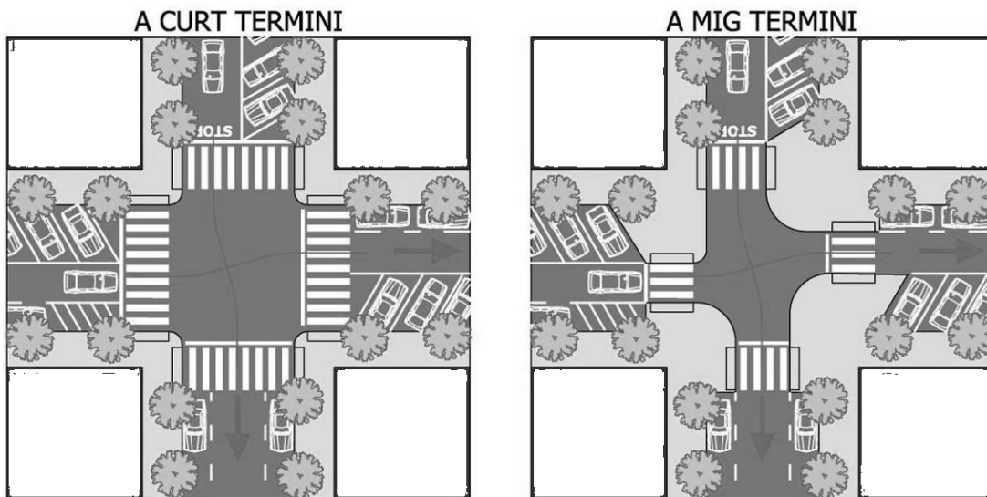
Figura 22. Aplicació de reductors horitzontals de velocitat a carrers amb calçades amples
