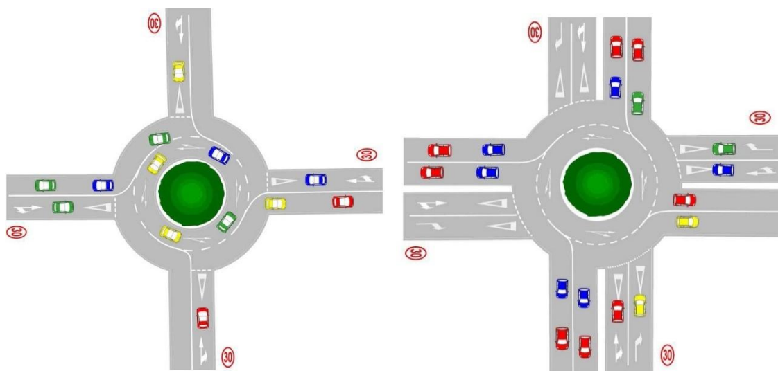
Figura 53. Proposta de senyalització en rotondes intel·ligents
