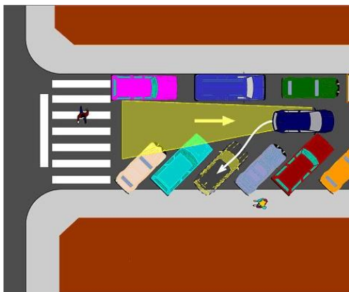
Figura 41. Sortida de semibateria amb visibilitat suficient
