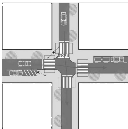
Figura 21. Aplicació de reductors horitzontals de velocitat a carrers d'entre 8 i 10 m
