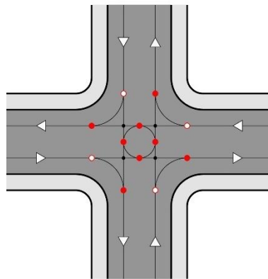
Figura 25. Punts de conflicte en una intersecció en X de doble sentit circulatori
