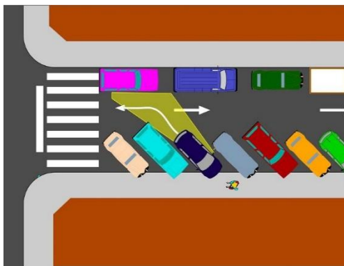
Figura 39. Sortida semibateria amb visibilitat insuficient
