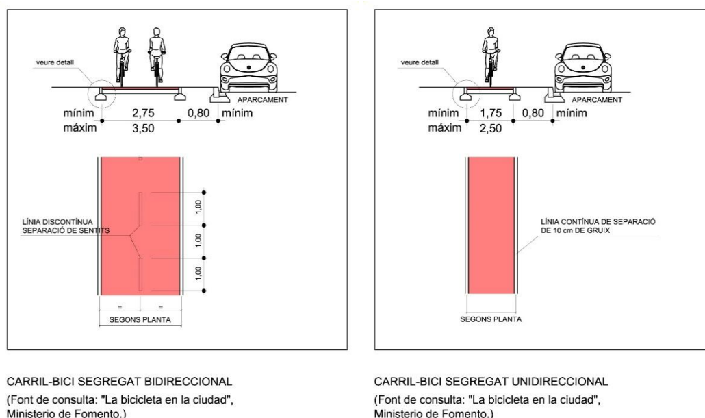
Figura 46. Dimensionament mínim per carrils bicicleta
