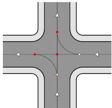
Figura 27. Punts de conflicte en una intersecció en X de sentit únic circulatori
