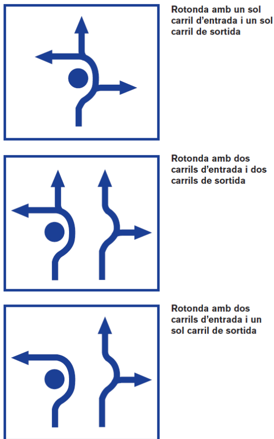
Figura 54. Proposta de fletxes de direcció prèvies a la rotonda
