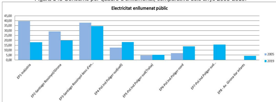
Figura 145 Consums per quadre d'enllumenat, comparativa dels anys 2005-2019.
