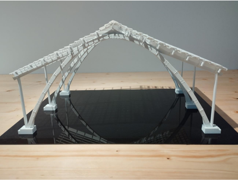
Antoni Gaudí. Nau de blanqueig de cotó, 1883 Maqueta de tres arcs amb detall del procés constructiu Impressió 3D amb filament de PLC 65,68 x 48,07 x 29,92 cm
