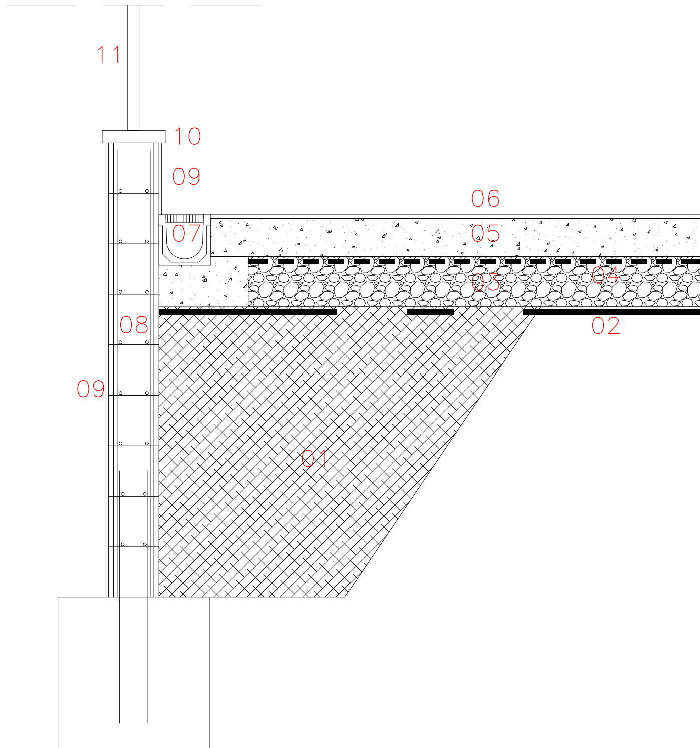
SECCIÓ CONSTRUCTIVA E=1/15
